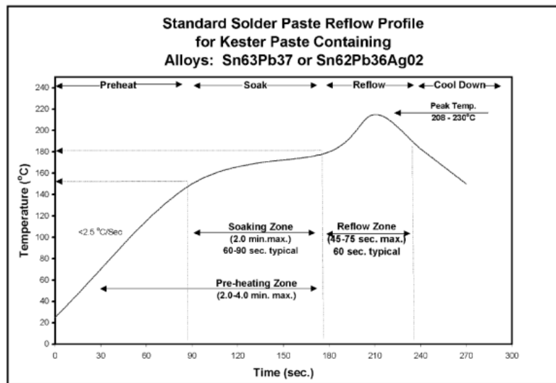
図 4 : はんだメーカーの推奨温度プロファイル J-STD-020
